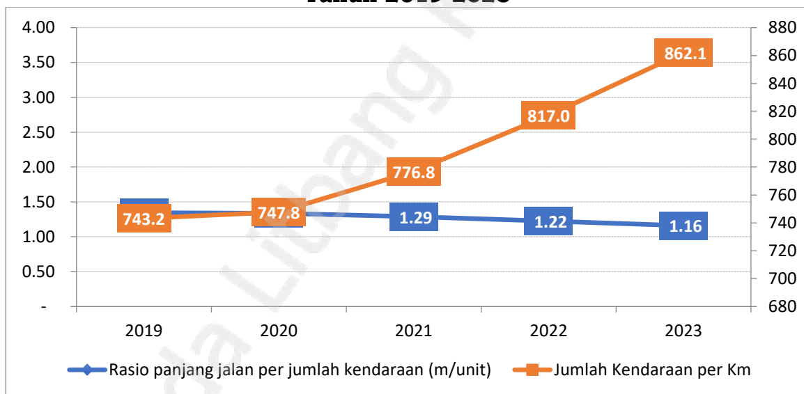
Gambar 2.35 Rasio Panjang Jalan per Jumlah Kendaraan Kota Tarakan Tahun 2019-2023
